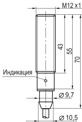
Габаритный чертеж
