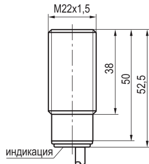
Габаритный чертеж
