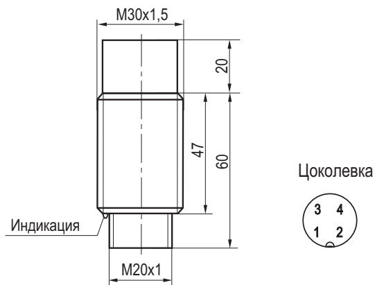
Габаритный чертеж
