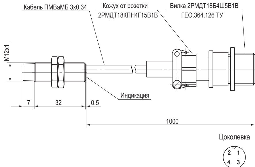
Габаритный чертеж
