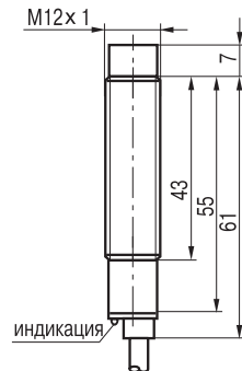
Габаритный чертеж
