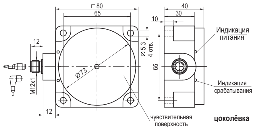
Габаритный чертеж
