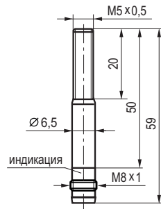
Габаритный чертеж
