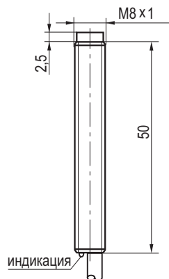
Габаритный чертеж
