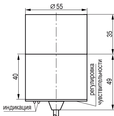
Габаритный чертеж
