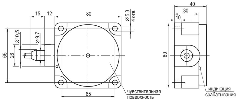
Габаритный чертеж
