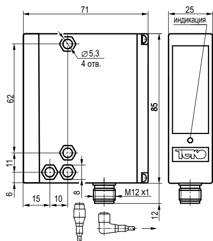
Габаритный чертеж.
