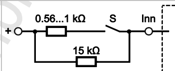
图：输入端 Inn 非电子开关 S
