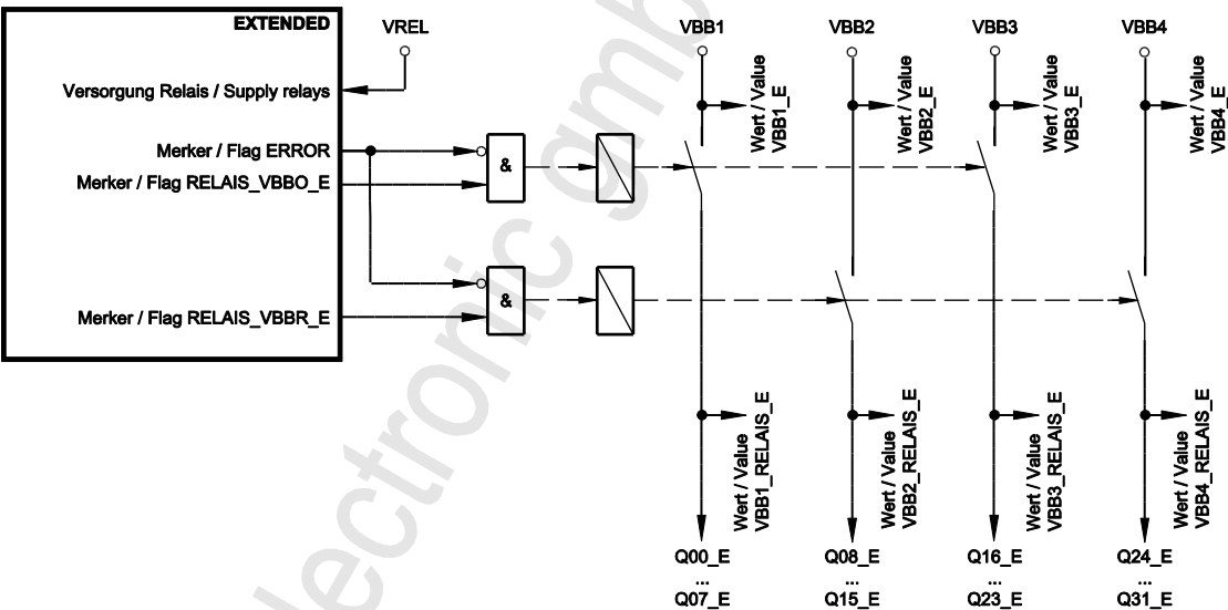
图：电源和继电器原理方块图（扩展侧）
