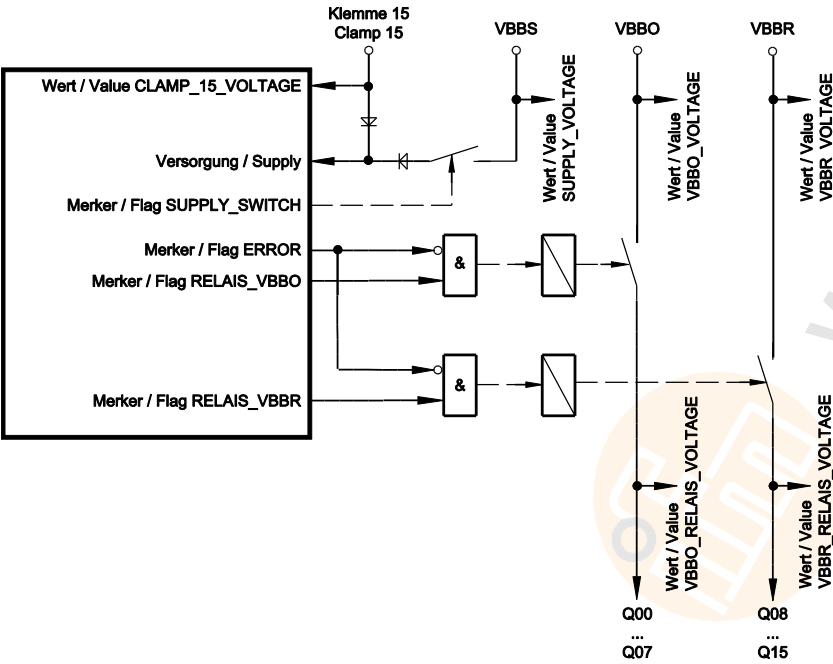
图：电源和继电器原理方块图（标准侧）
