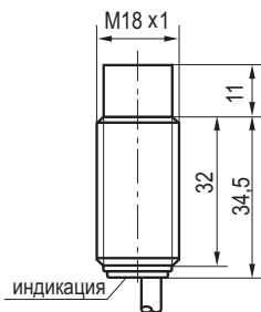
Габаритный чертеж
