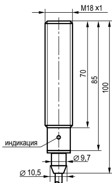
Габаритный чертеж.
