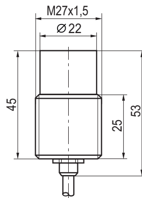
Габаритный чертеж
