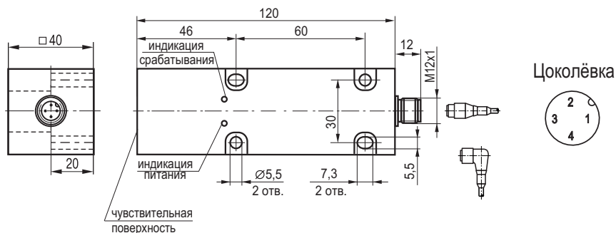
Габаритный чертеж
