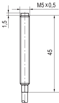
Габаритный чертеж
