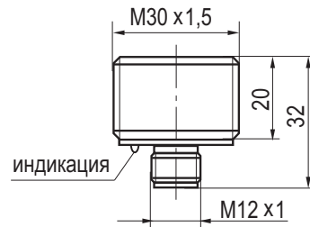
Габаритный чертеж
