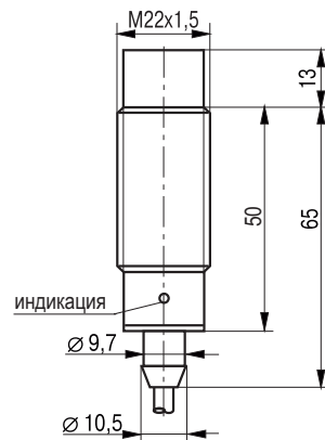
Габаритный чертеж
