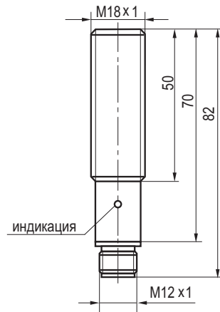
Габаритный чертеж
