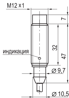
Габаритный чертеж
