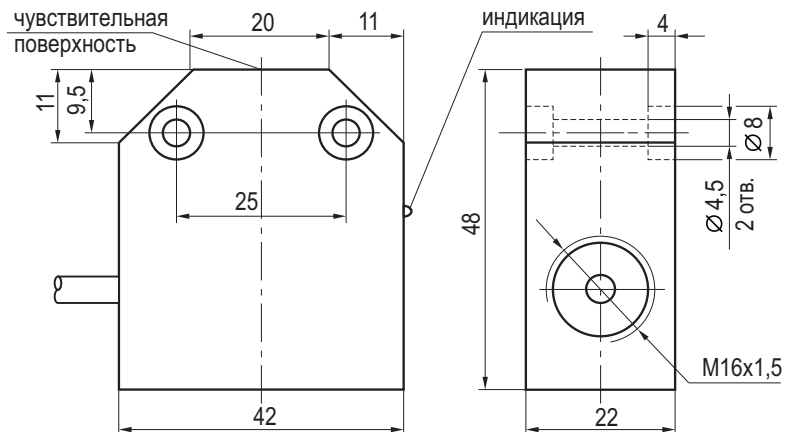
Габаритный чертеж
