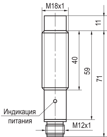
Габаритный чертеж
