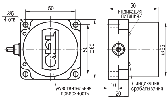
Габаритный чертеж
