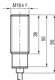
Габаритный чертеж
