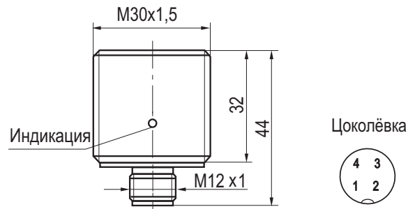
Габаритный чертеж
