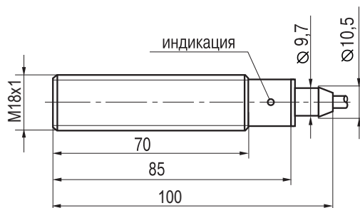
Габаритный чертеж
