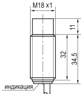
Габаритный чертеж
