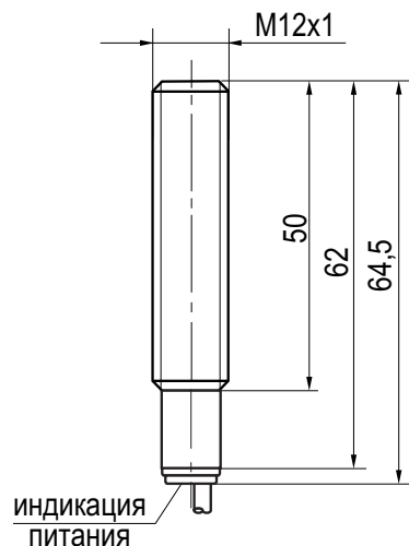
Габаритный чертеж
