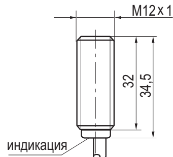
Габаритный чертеж
