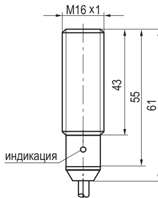
Габаритный чертеж
