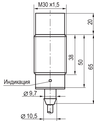
Габаритный чертеж
