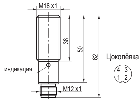
Габаритный чертеж
