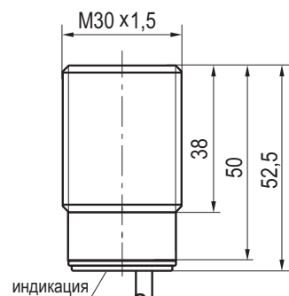
Габаритный чертеж
