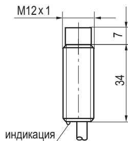
Габаритный чертеж
