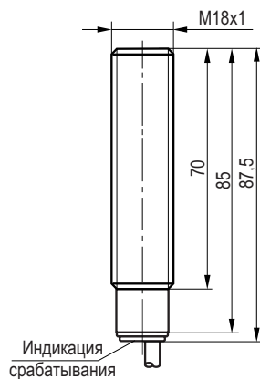
Габаритный чертеж
