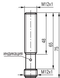
Габаритный чертеж
