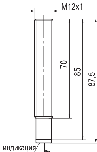
Габаритный чертеж
