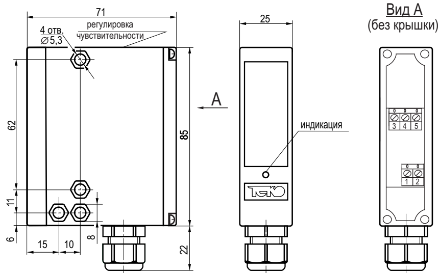
Габаритный чертёж.
