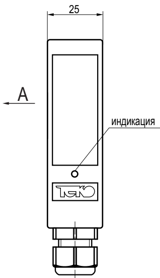
Габаритный чертеж.
