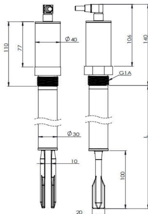
Размеры, мм
