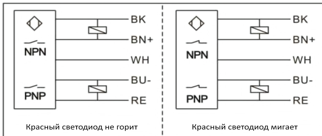
Схема подключения
