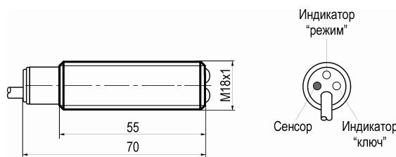
Рисунок 1 - Габаритный чертёж
