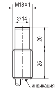
Габаритный чертеж
