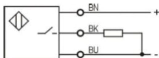
PNP NO
