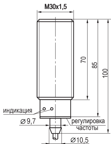
Габаритный чертеж
