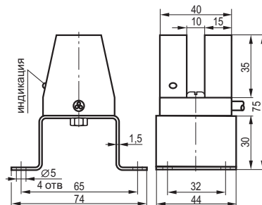
Габаритный чертеж
