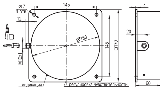
Габаритный чертеж
