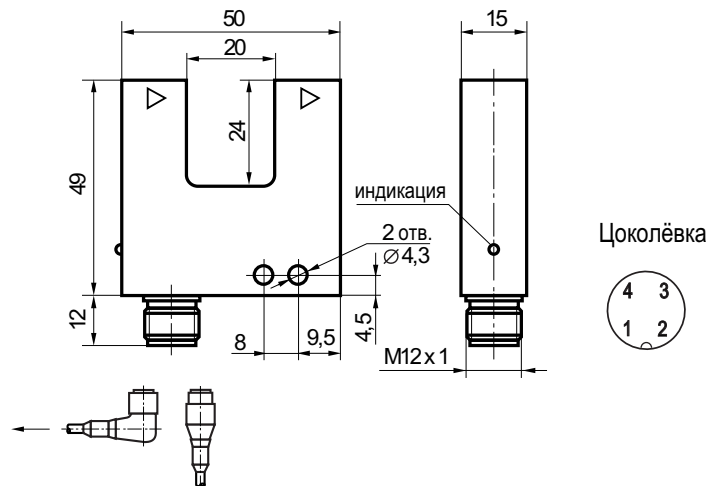
Габаритный чертеж
