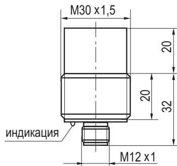
Габаритный чертеж
