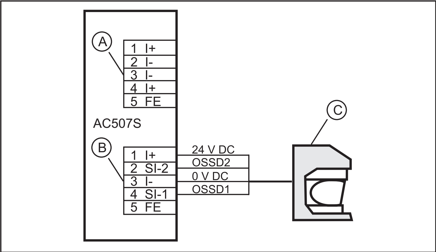
A: socket 3 / B: socket 1 / C: laser scanner
